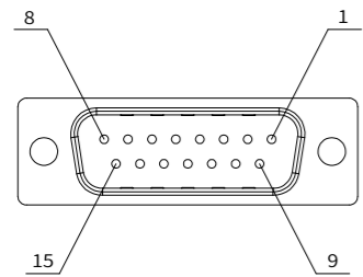
DB15母头
